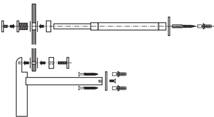
Montaje con paneles de vidrio
