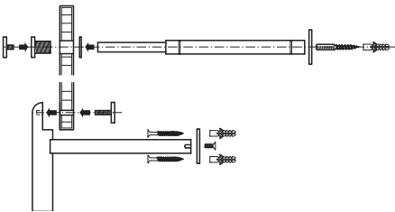
Montaje con paneles de madera
